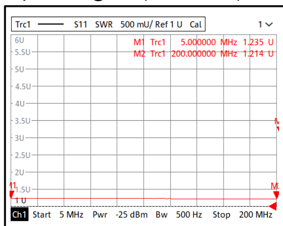
Input VSWR @+85°C (5MHz-200MHz)
