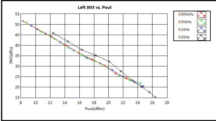
Left IM3 vs. Pout (5MHz-200MHz)
