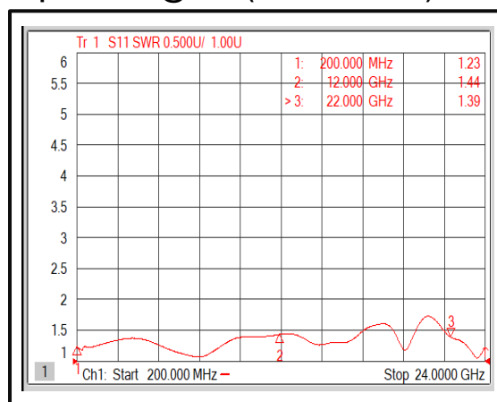
Input VSWR @-40°C (200MHz-22GHz)
