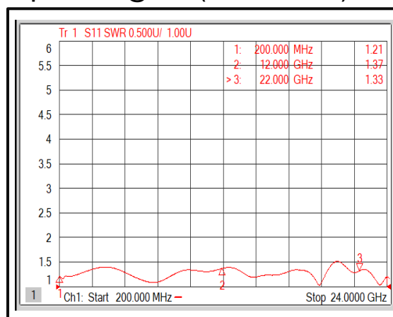
Input VSWR @+85°C (200MHz-22GHz)
