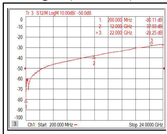
Isolation@-40°C (200MHz-22GHz)
