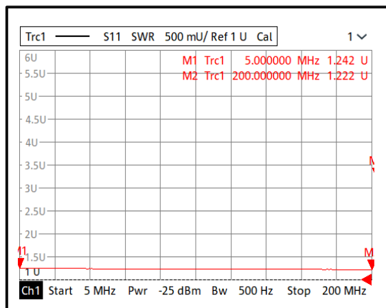
Input VSWR @+25°C (5MHz-200MHz)
