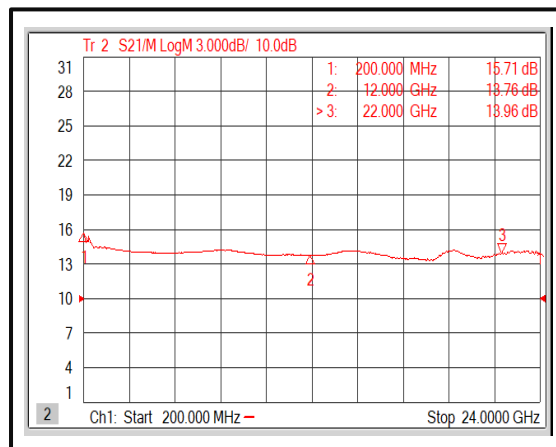
Gain@-40°C (200MHz-22GHz)
