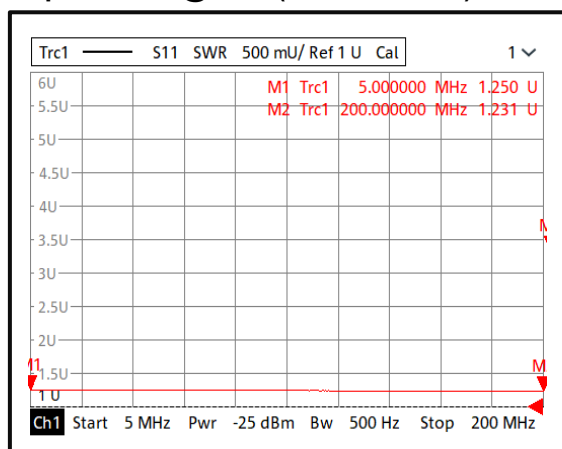
Input VSWR @-40°C (5MHz-200MHz)
