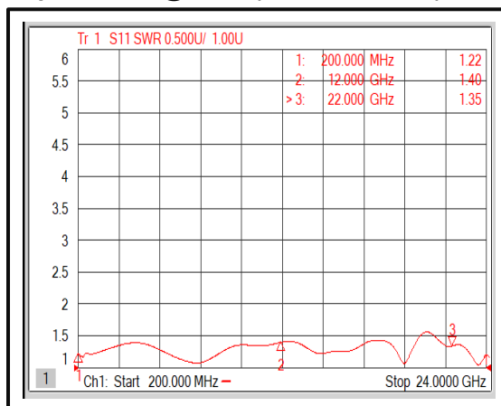
Input VSWR @+25°C (200MHz-22GHz)
