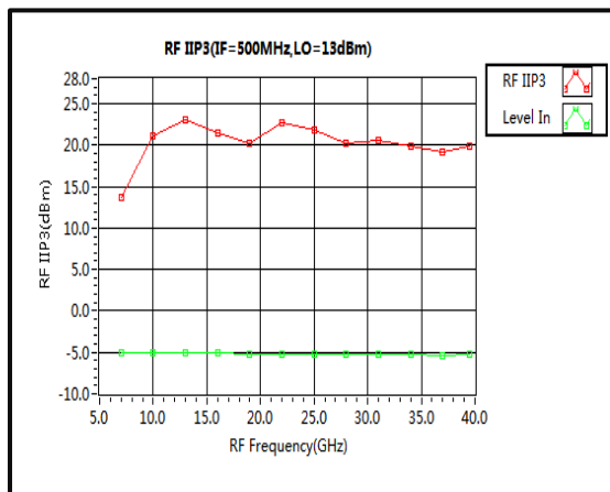
RF IIP3
