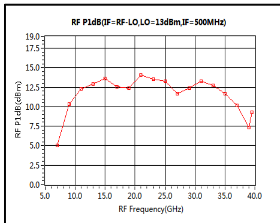
RF P1dB
