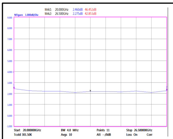
Noise Figure(20-26.5GHz)
