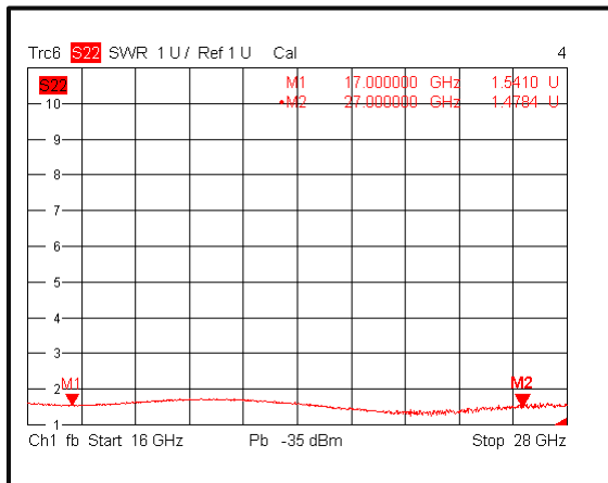
Output VSWR@-40°C
