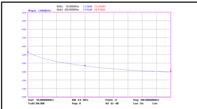
Noise Figure(50MHz-200MHz)
