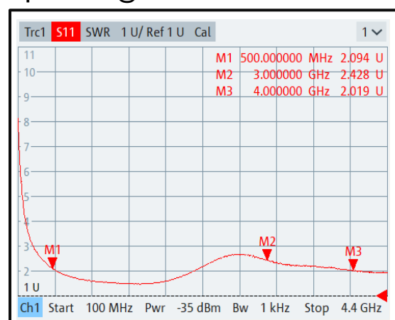
Input VSWR@+85°C
