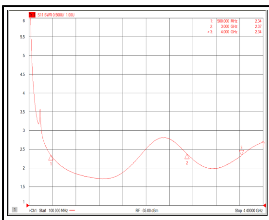
Input VSWR@+85°C
