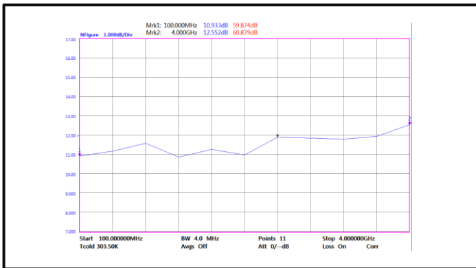
Noise Figure(100MHz-4GHz)
