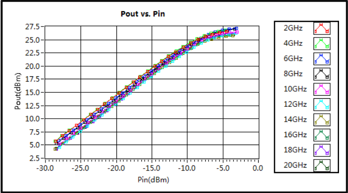
Pout vs.Pin
