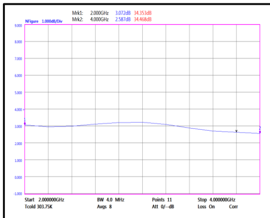
Noise Figure(2GHz-4GHz)
