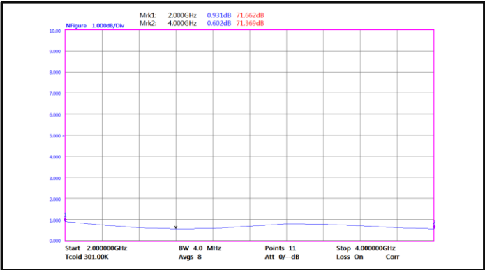
Noise Figure(2GHz-4GHz)
