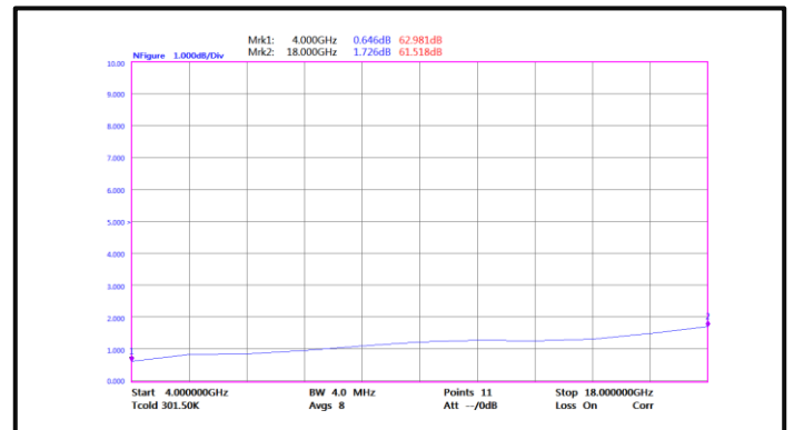
Noise Figure(4GHz-18GHz)
