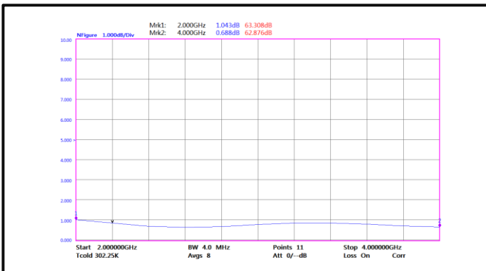
Noise Figure(2GHz-4GHz)
