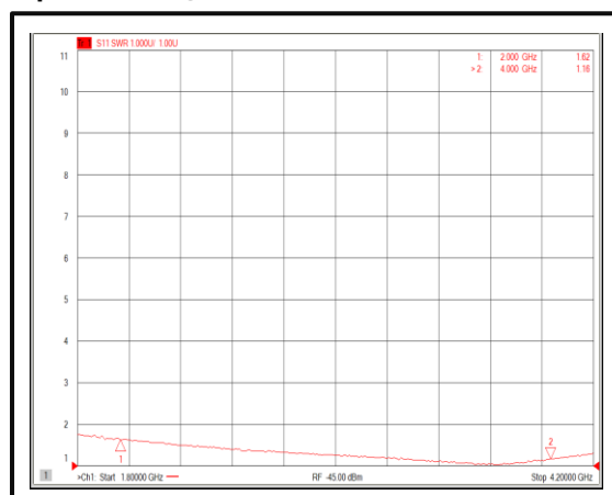
Input VSWR@+85°C
