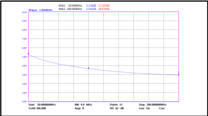
Noise Figure(50MHz-200MHz)
