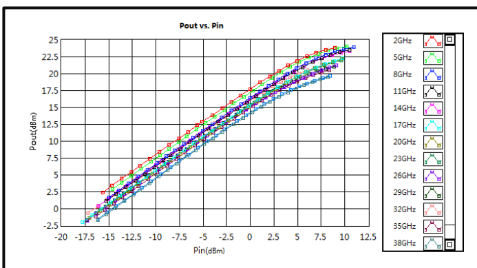
Pout vs. Pin (2GHz-38GHz)
