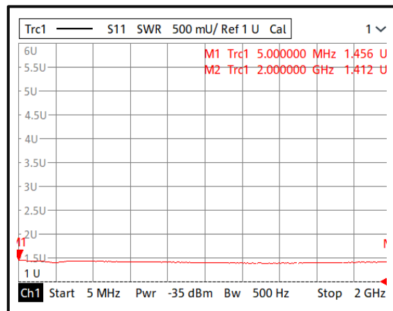
Input VSWR@+85°C (0.005-2GHz)
