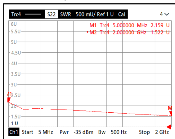
Output VSWR@+85°C (0.005-2GHz)
