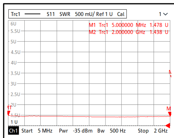
Input VSWR@-40°C (0.005-2GHz)
