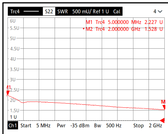
Output VSWR@-40°C (0.005-2GHz)
