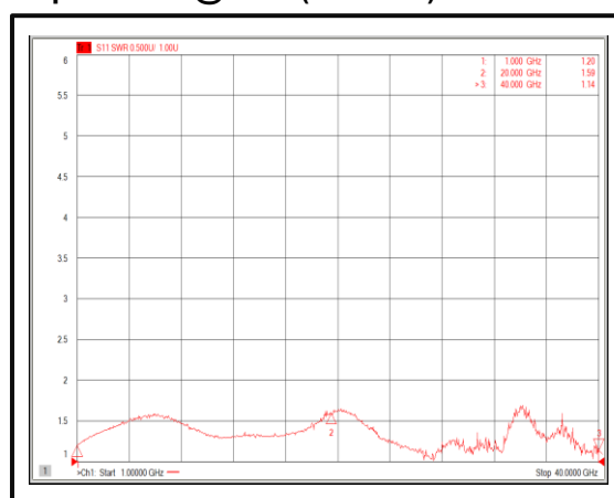
Input VSWR@-40°C (1-40GHz)
