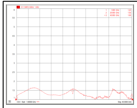
Input VSWR@+85°C (1-40GHz)
