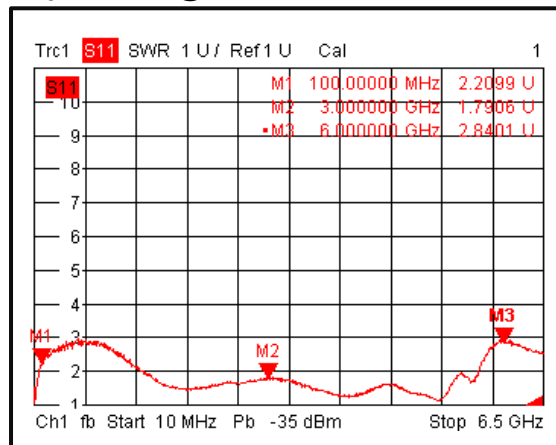
Input VSWR@+85°C
