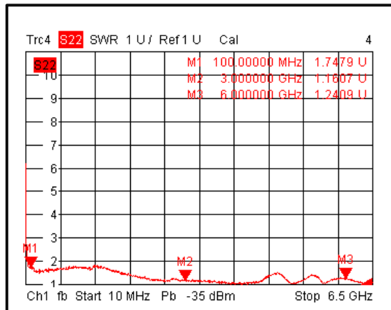
Output VSWR@-40°C
