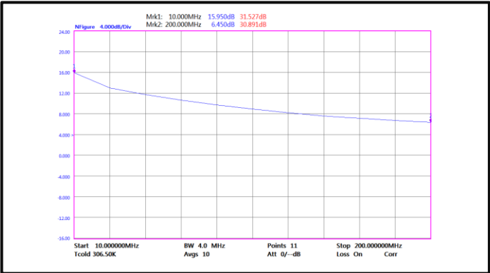
Noise Figure(0.01-0.2GHz)
