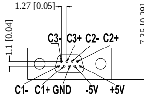
MICRO-D9(Female)
