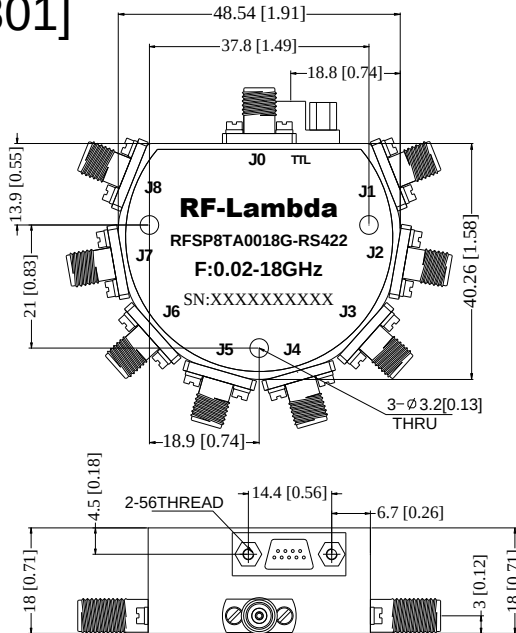
MICRO-D9(Female)
