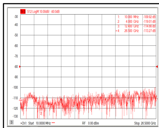
Isolation @+75°C
