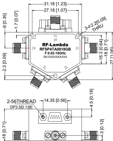
MICRO-D9(Female)
