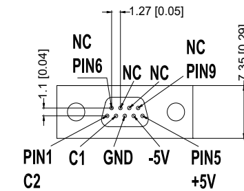
MICRO-D9(Female)
