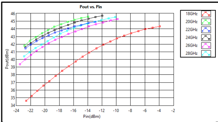
Output vs Input Power CW (18-28GHz)
