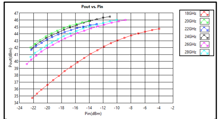
Output vs Input Power *Pulse (18-28GHz)
