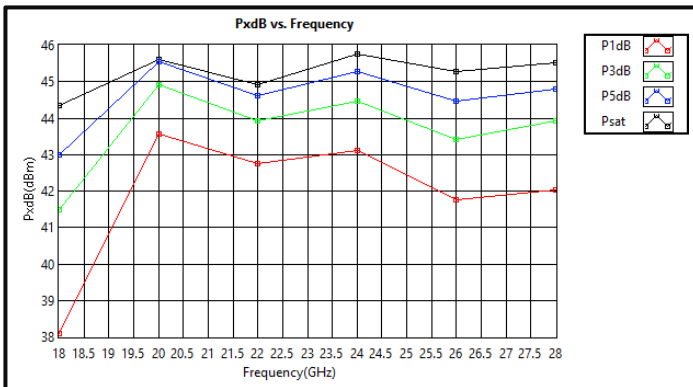
PxdB vs Frequency CW (18-28GHz)
