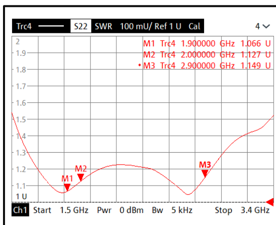
VSWR 2
