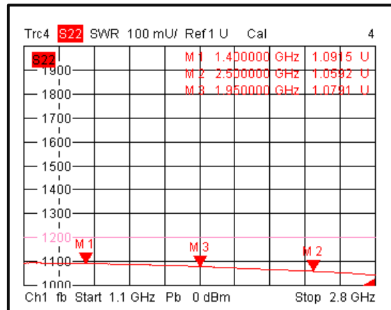
Output VSWR
