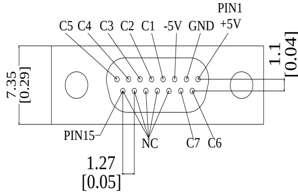
MICRO-D15(Female)
