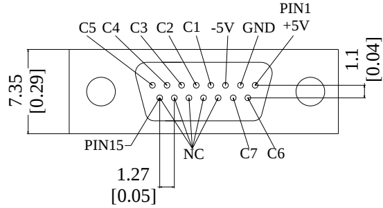
MICRO-D15(Female)
