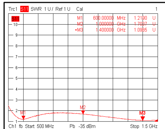
Input VSWR@-40°C
