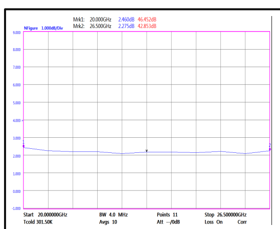
Noise Figure(20-26.5GHz)
