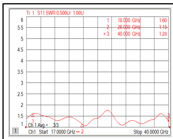
Input VSWR @-30°C
