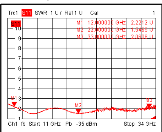
Input VSWR@-40°C
