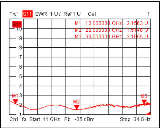
Input VSWR@+25°C
