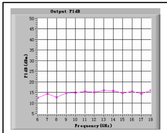
Output P1dB
