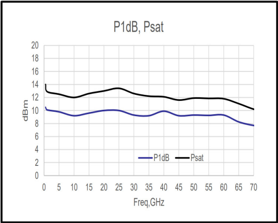
Psat & P1dB
