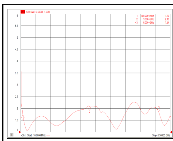
Input VSWR@-40°C
