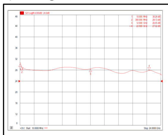
Input VSWR@-40°C
