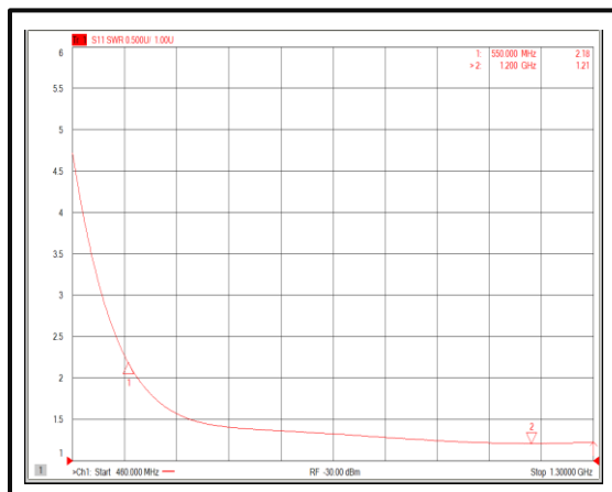
Input VSWR@-40°C (+5V)
