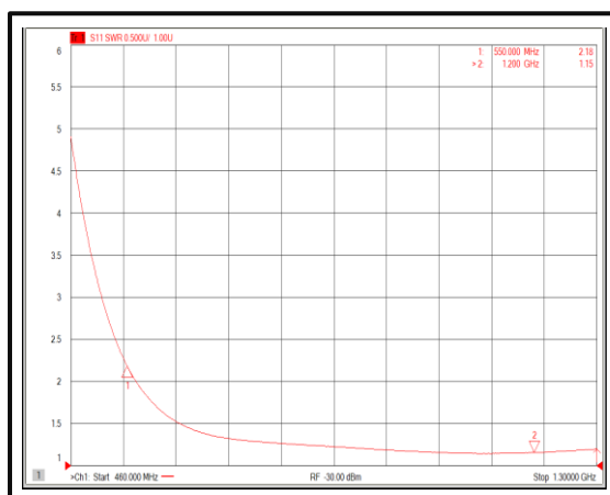
Input VSWR@+85°C (+5V)
