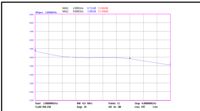
Noise Figure(2GHz-4GHz)
