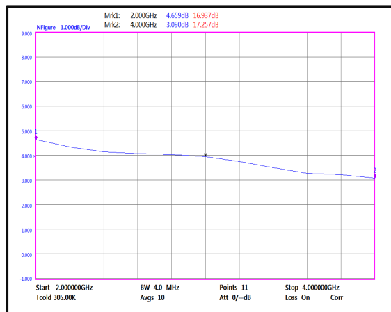
Noise Figure(2GHz-4GHz)
