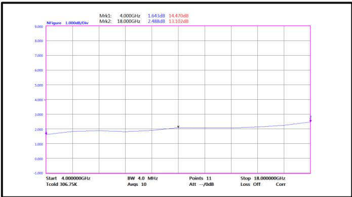
Noise Figure(4GHz-18GHz)
