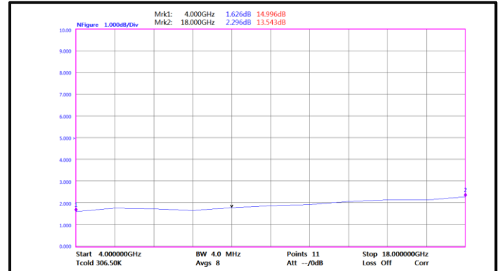
Noise Figure(4GHz-18GHz)
