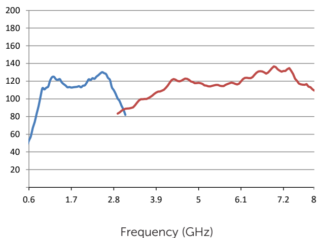
VSWR Lo/Hi
